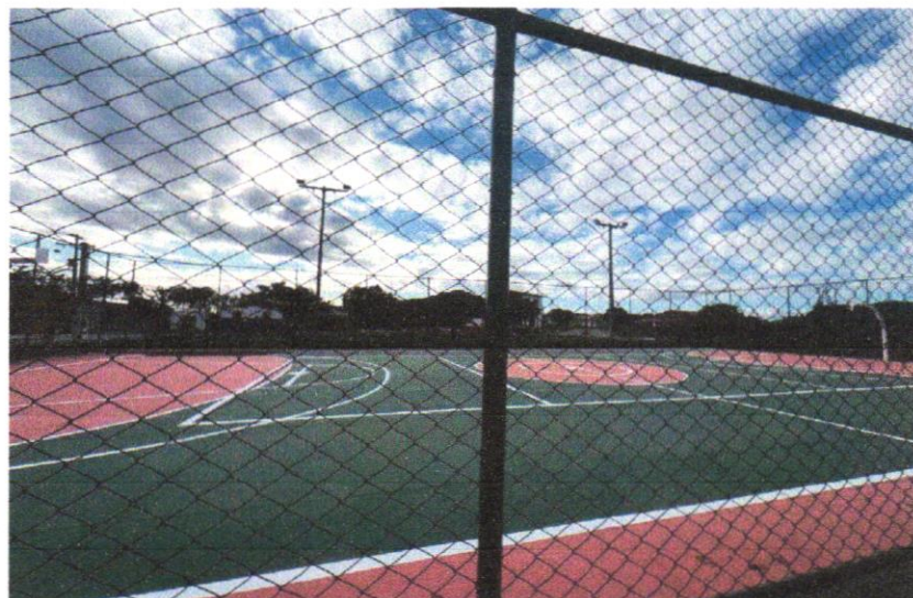
FOTO 06 - ALAMBRADO PARA QUADRA POLIESPORTIVA, ESTRUTURADO POR TUBOS DE ACO GALVANIZADO, (MONTANTES COM DIAMETRO 2", TRAVESSAS E ESCORAS COM DIÂMETRO 1 ¼ ), COM TELA DE ARAME GALVANIZADO, FIO 10 BWG E MALH
