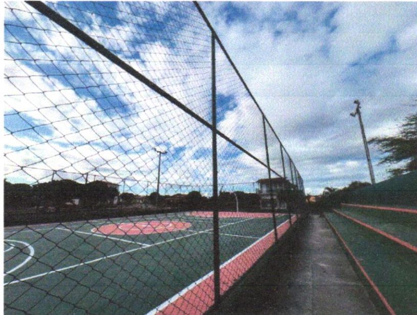
FOTO 05 - ALAMBRADO PARA QUADRA POLIESPORTIVA, ESTRUTURADO POR TUBOS DE ACO GALVANIZADO, (MONTANTES COM DIAMETRO 2", TRAVESSAS E ESCORAS COM DIÂMETRO 1 ¼ ), COM TELA DE ARAME GALVANIZADO, FIO 10 BWG E MALHA
