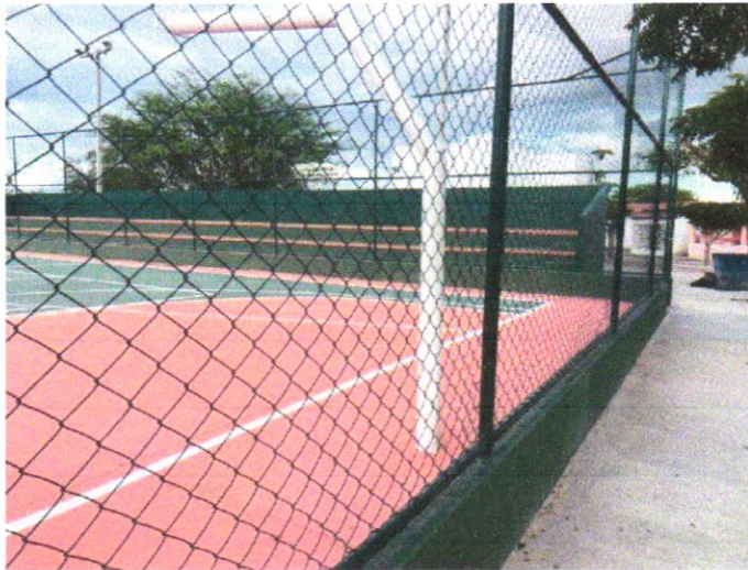
FOTO 03 - ALAMBRADO PARA QUADRA POLIESPORTIVA, ESTRUTURADO POR TUBOS DE ACO GALVANIZADO, (MONTANTES COM DIAMETRO 2", TRAVESSAS E ESCORAS COM DIÂMETRO 1 ¼ ), COM TELA DE ARAME GALVANIZADO, FIO 10 BWG E MALHA
